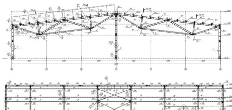
ГАБАРИТЫ ЗДАНИЯ
