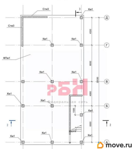
Схема расположения конструкций на отм. -0,000
