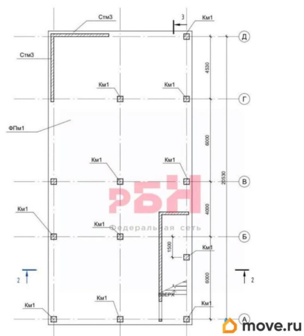
Схема расположения конструкций на отм. -0,000
